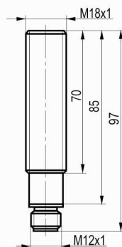
Габаритный чертеж
